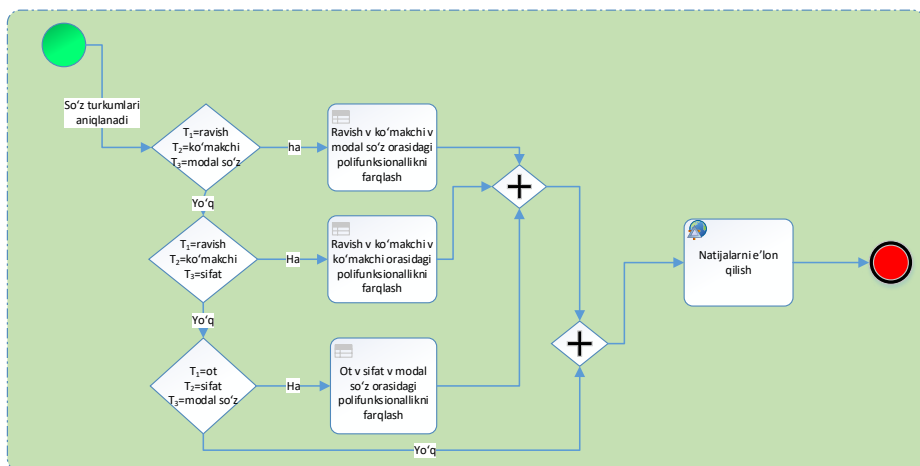
5-rasm: Uchta soʻz turkumi doirasidagi polifunksionallikni farqlovchi biznes-jarayon modeli
