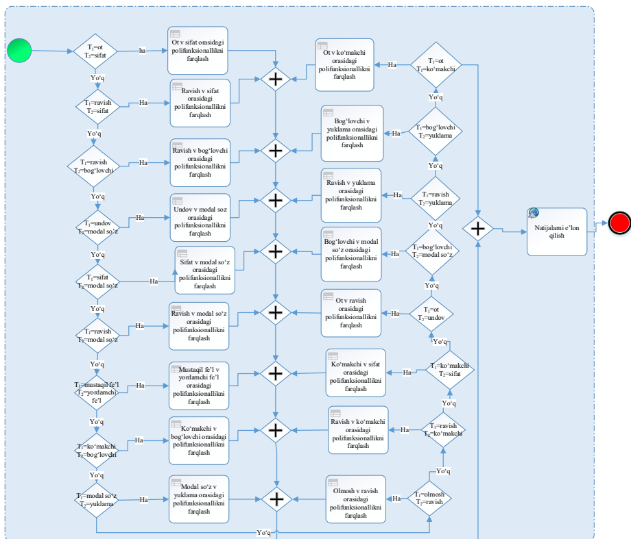
4-rasm: Ikkita soʻz turkumi doirasidagi polifunksionallikni farqlovchi biznes-jarayon modeli
